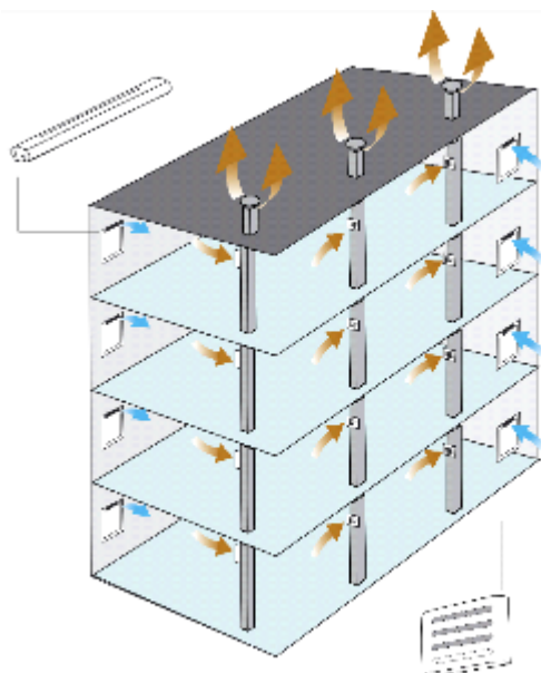
Image : système de ventilation hygroréglable complet.
